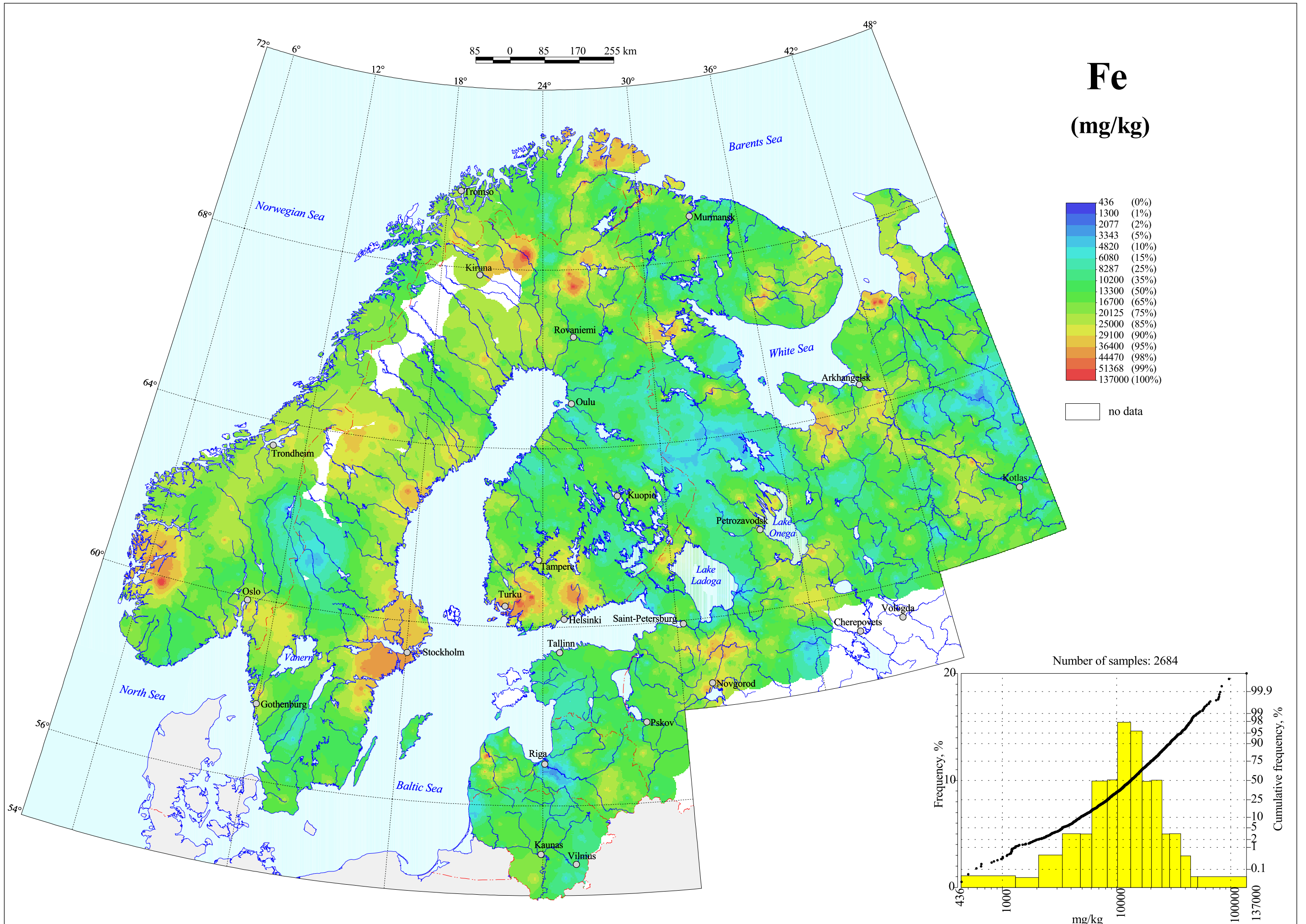
Iron in C-horizon, Grain Size <2 mm, Aqua regia Extraction
